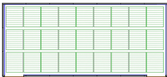
FN-7: 8,40 m x 3,72 m x 2,58 m 27 carros de 1,00m x 0,80m 40 carros de 0,90 m x 0,60 m
