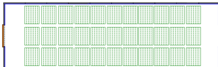
FN-9: 12,00 m x 3,73 m x 2,58 m 30 carros de 1,00 m x 0,80 m
