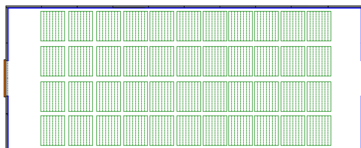
FN-10: 12,00 m x 4,80 m x 3,00 m 40 carros de 1,00m x 0,80 m
