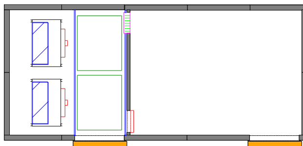
TM-4: 5,80 m x 2,60 m x 2,60 m Capacidad congelación: 75 kg/h Almacenamiento: 150 cajas de 0,6x0,4x0,3 m
