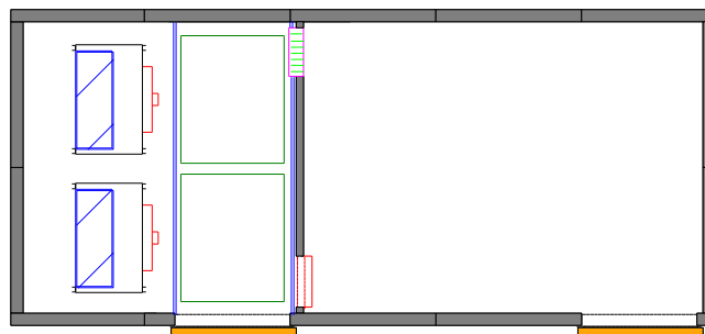
TMD-3: 5,80 m x 2,60 m x 2,60 m Capacidad congelación: 75 kg/h Almacenamiento: 150 cajas de 0,6x0,4x0,3 m
